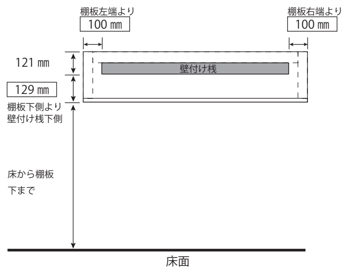
■壁付け桟取付寸法図
