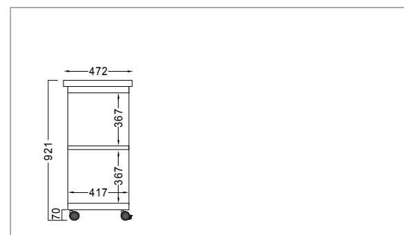
■AW-90C 側面図
