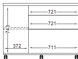
■AW-90W 側面図
