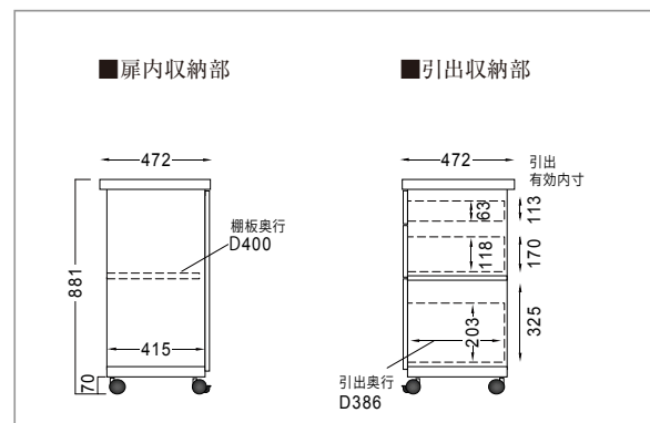
■CW-90W 側面図
