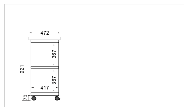
■CW-90C 側面図
