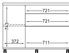
■CW-90W 側面図
