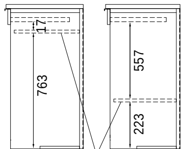
■オープン部内の可動棚詳細 (602K・S602K)
