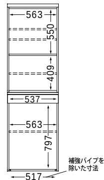
■オープン部内の可動棚詳細 (602K・S602K)
