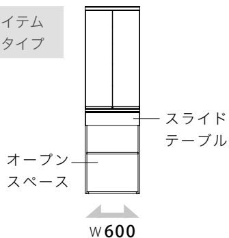
テーブル付 スリムストッカー
