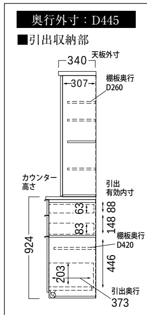
■共通側面図 (S601K)
