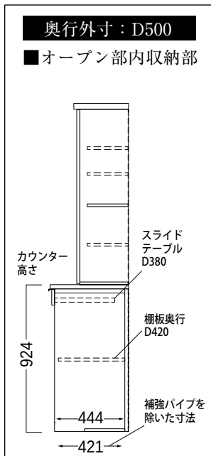
■共通側面図 (602K)
