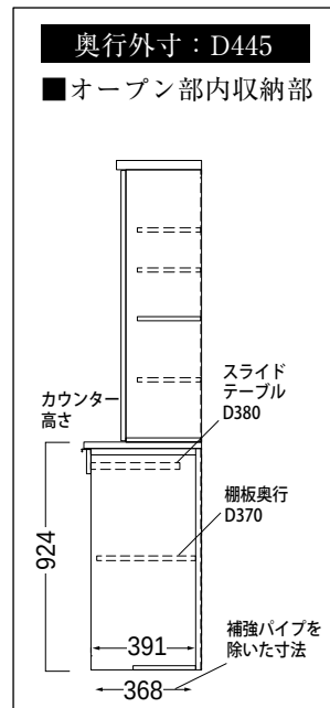
■共通側面図 (S602K)
