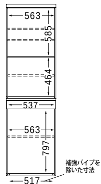
■オープン部内の可動棚詳細 (602K・S602K)
