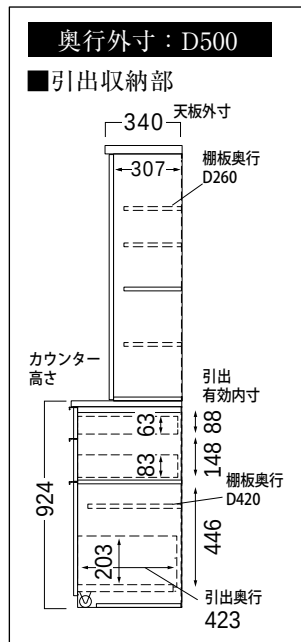
■共通側面図 (601K)
