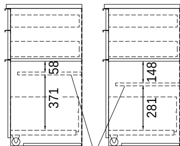
■引出内の可動棚詳細 (601K・S601K)
