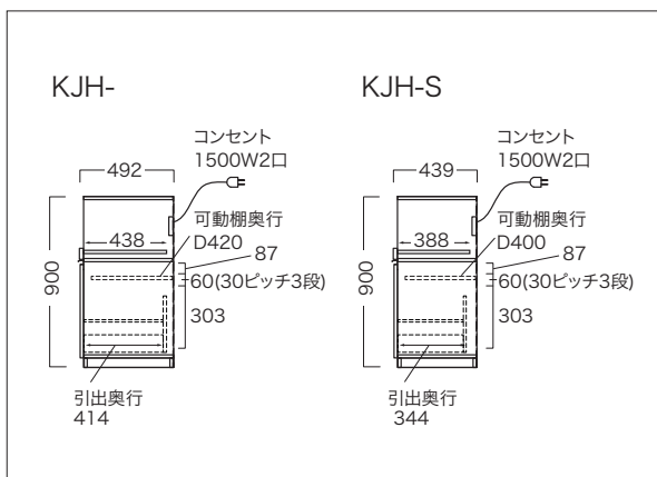
◎共通側面図
