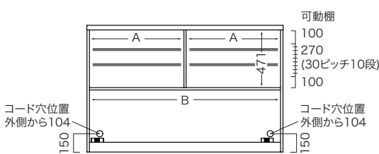
■正面図
