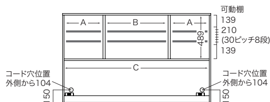
■正面図
