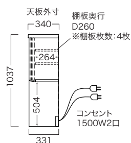
◎共通側面図
