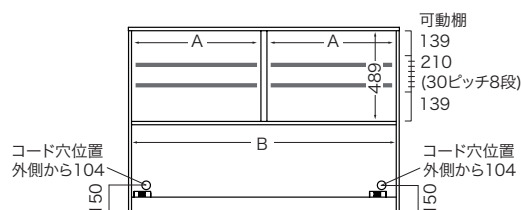
■正面図
