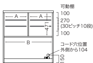
■正面図
