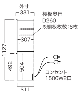
◎共通側面図
