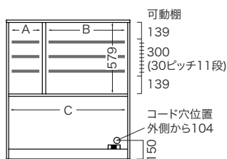
■正面図
