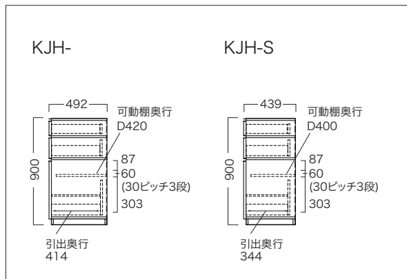
◎共通側面図
