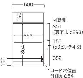
■正面図
