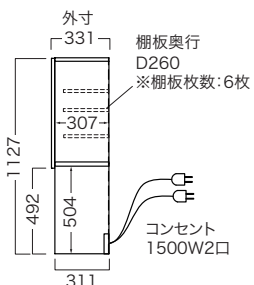
◎共通側面図
