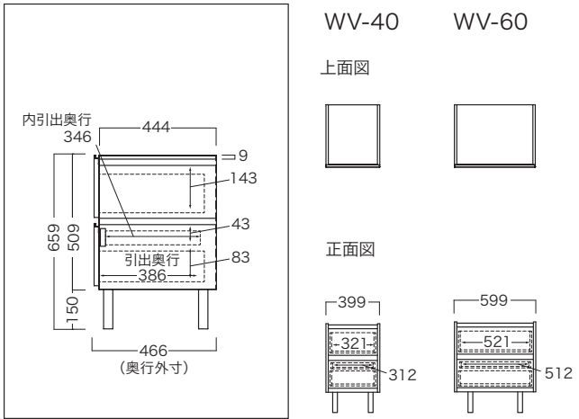
◎共通側面図 (WV-40／60)
