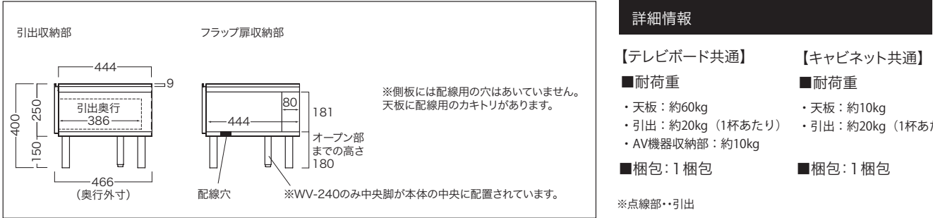
◎共通側面図 (WV-150～240)
