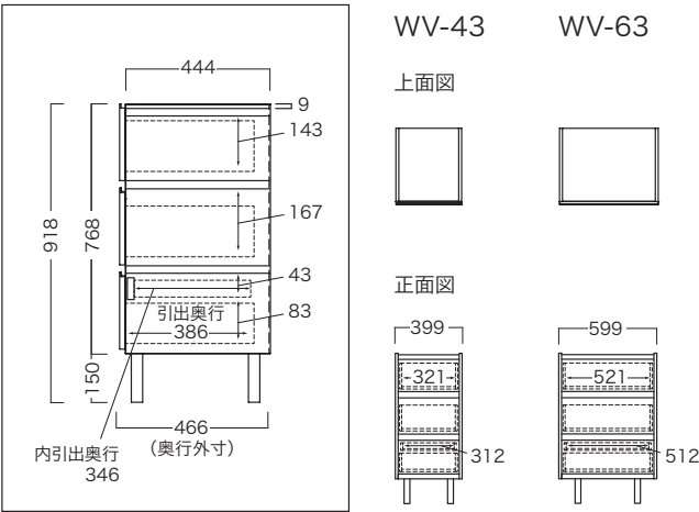
◎共通側面図 (WV-43／63)
