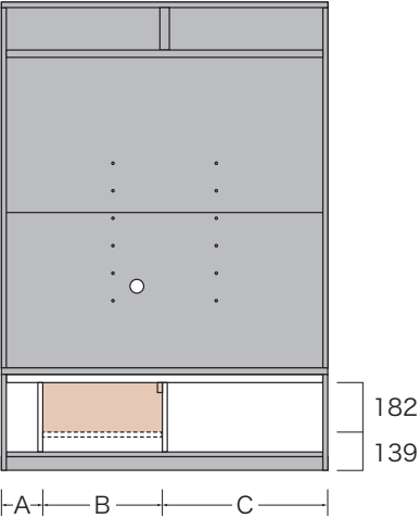
正面図（構造図）
