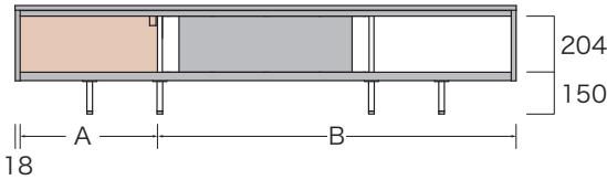
正面図（構造図）
