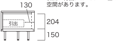
側面図
