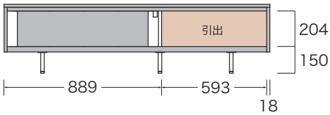
正面図（構造図）
