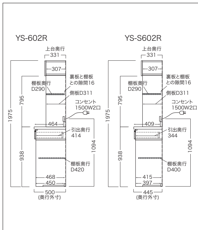
側面図
