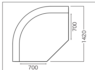
PY-CR上面図
