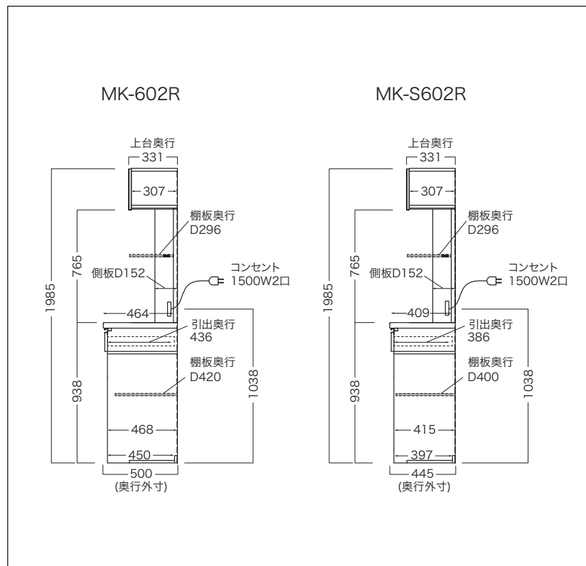
側面図
