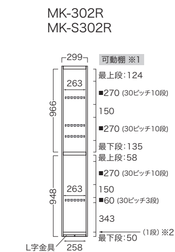
正面図
