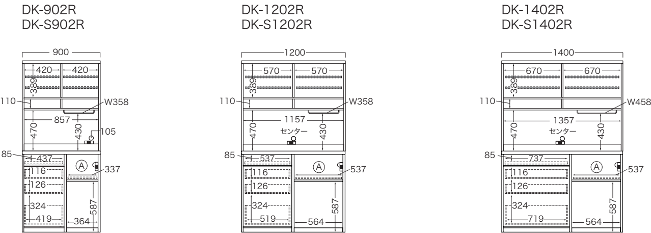
正面図
