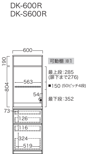
正面図
