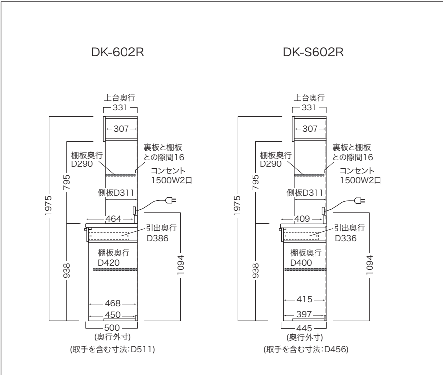
側面図
