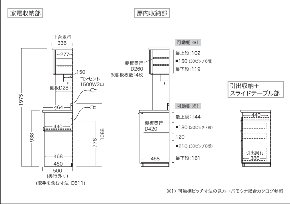
奥行外寸：D500 共通側面図 (DK-902R～1802R)
