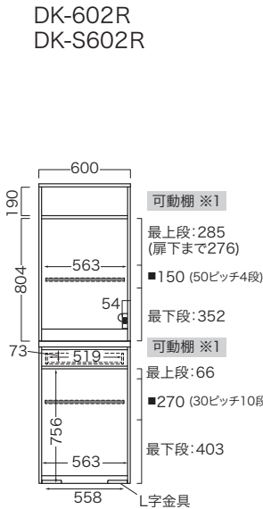
正面図
