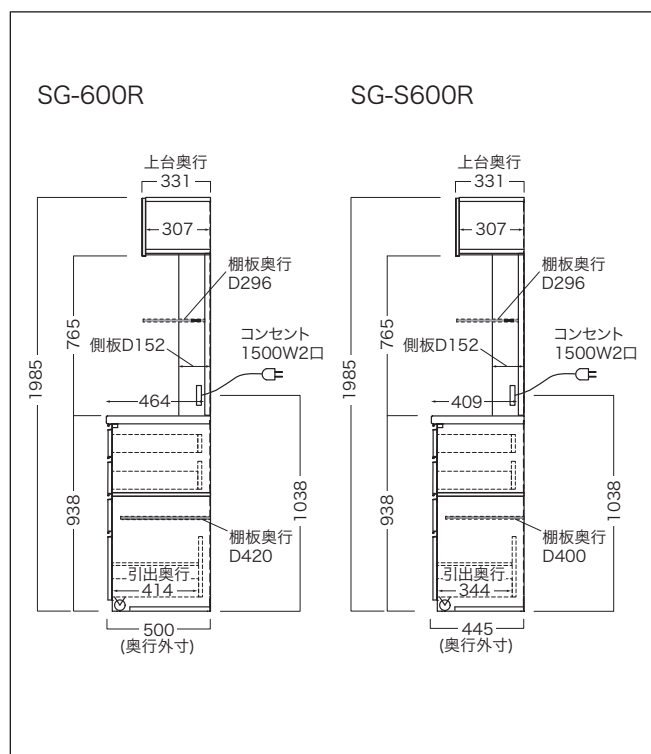
側面図
