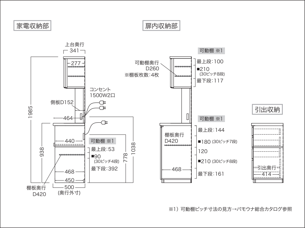
奥行外寸:D500 共通側面図(SG-1002R~1802R)
