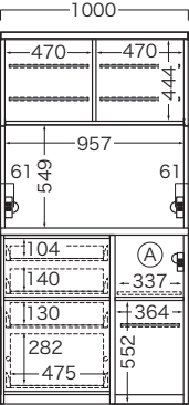
SG-1002R SG-S1002R
