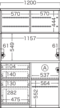
SG-1202R SG-S1202R
