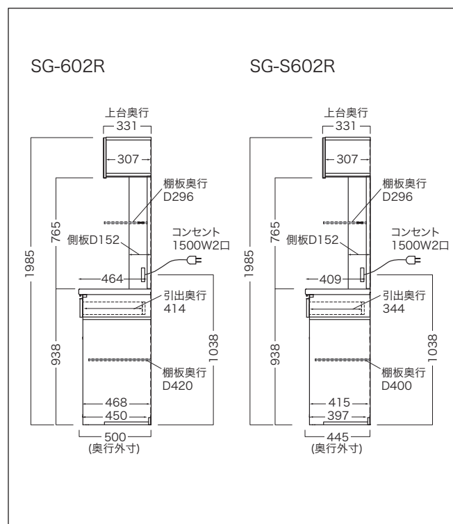
■家電タワー可動棚詳細(3段)
