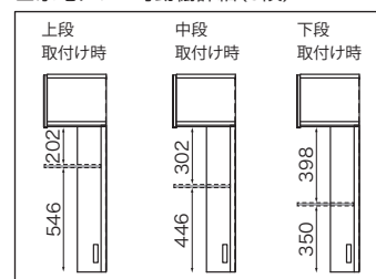
■家電タワー可動棚詳細(3段)
