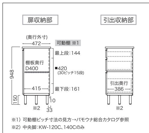
◎共通側面図 (KW-90C~140C)
